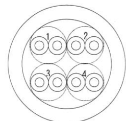
CAT-5e 配列図
